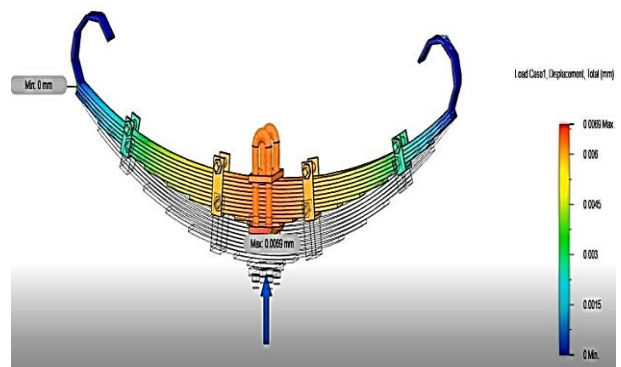
Fig. 27. Beryllium oxide displacement.
