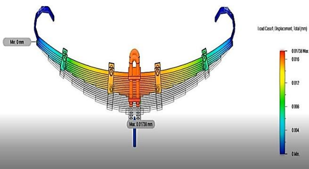
Fig. 21. Titanium alloy Displacement distribution.
